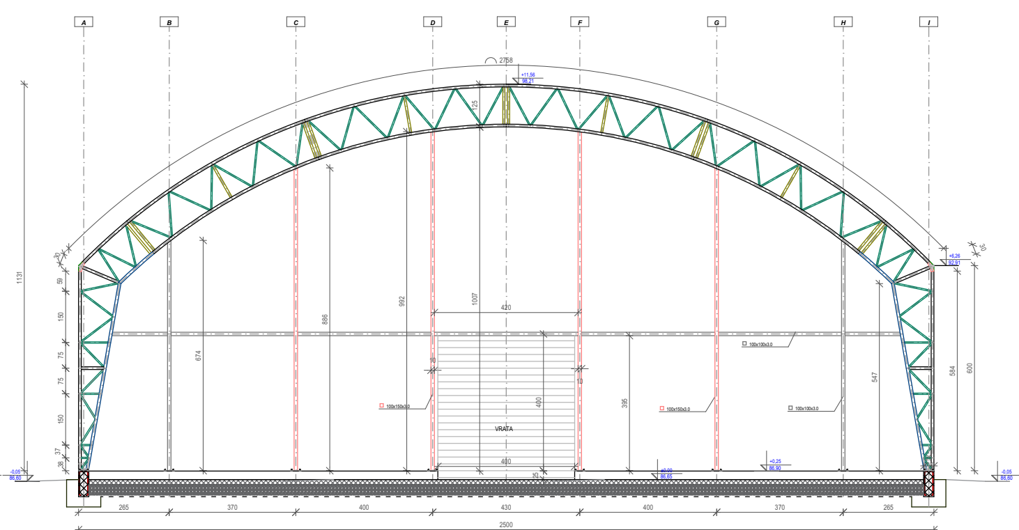
PRESEK A-A
