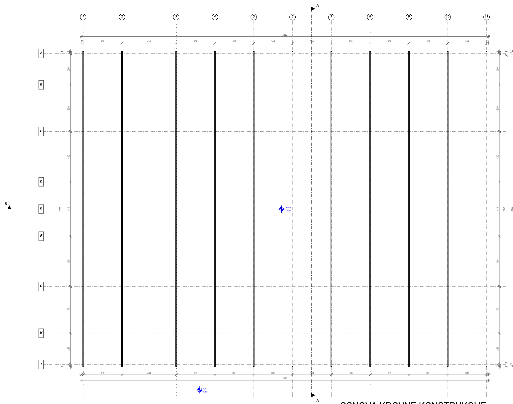
OSNOVA KROVNE KONSTRUKCIJE
