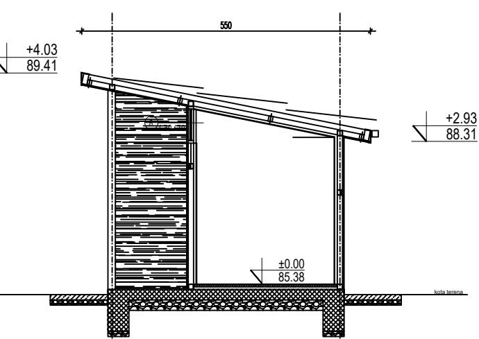
PRESEK A-A
