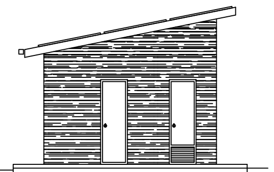
JUGOISTOČNA FASADA
