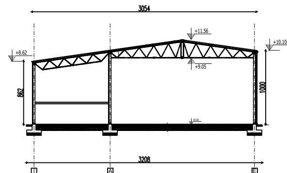
PRESEK A-A
