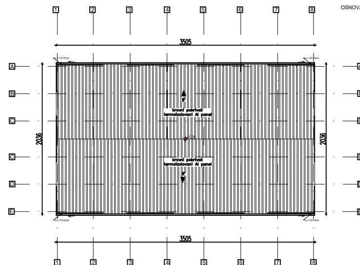
OSNOVA KROVNIH RAVNI
