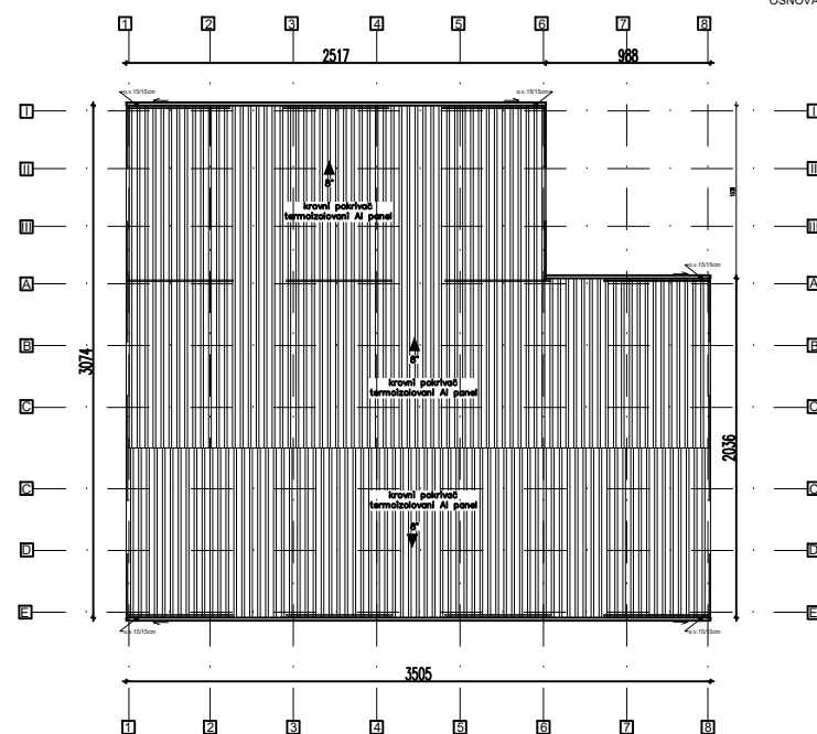
OSNOVA KROVNIH RAVNI
