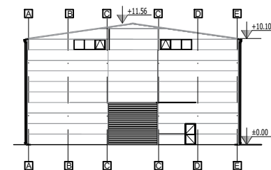
JUZNA FASADA
