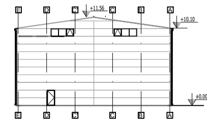
SEVERNA FASADA
