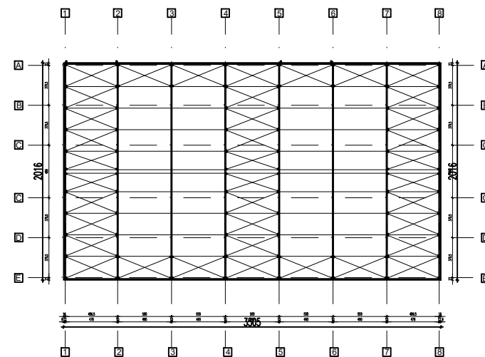
OSNOVA KROVNE KONSTRUKCIJE
