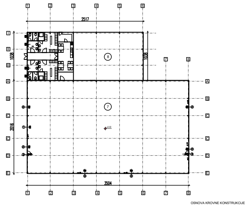
OSNOVA KROVNE KONSTRUKCIJE
