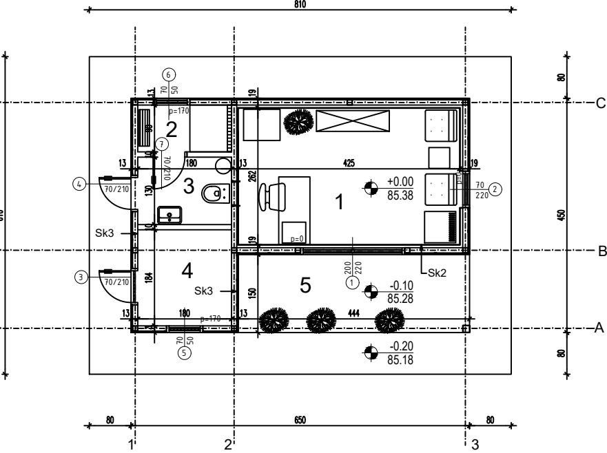
OSNOVA PRIZEMLJA
