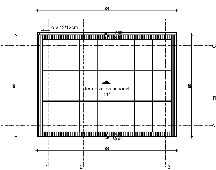
OSNOVA KROVNE RAVNI
