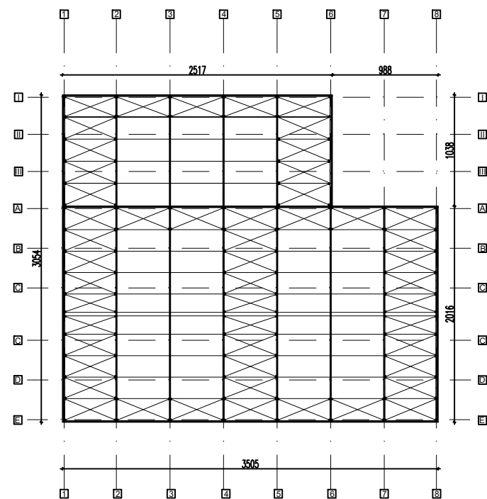
OSNOVA KROVNE KONSTRUKCIJE
