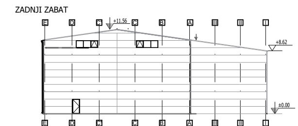
ZADNJI ZABAT
