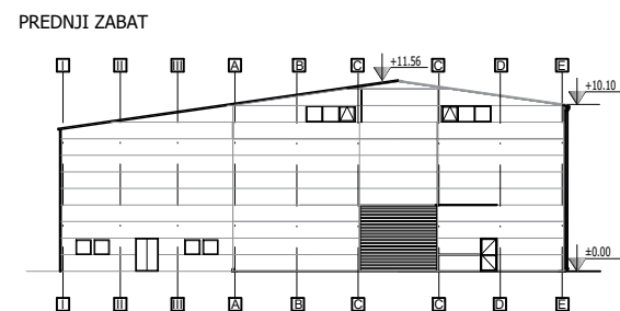
PREDNJI ZABAT
