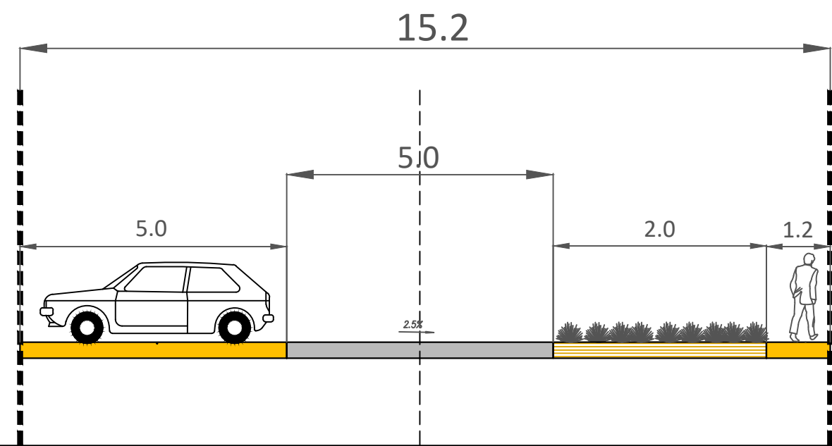
ПОПРЕЧНИ ПРОФИЛ 4-4
