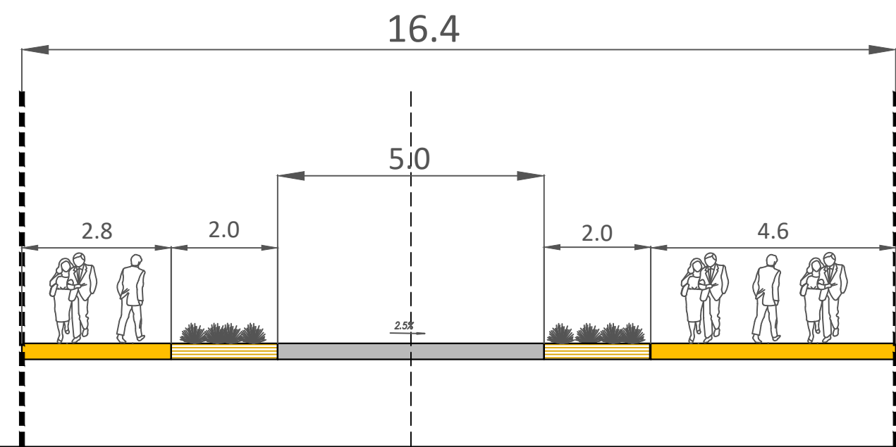
ПОПРЕЧНИ ПРОФИЛ 2-2
