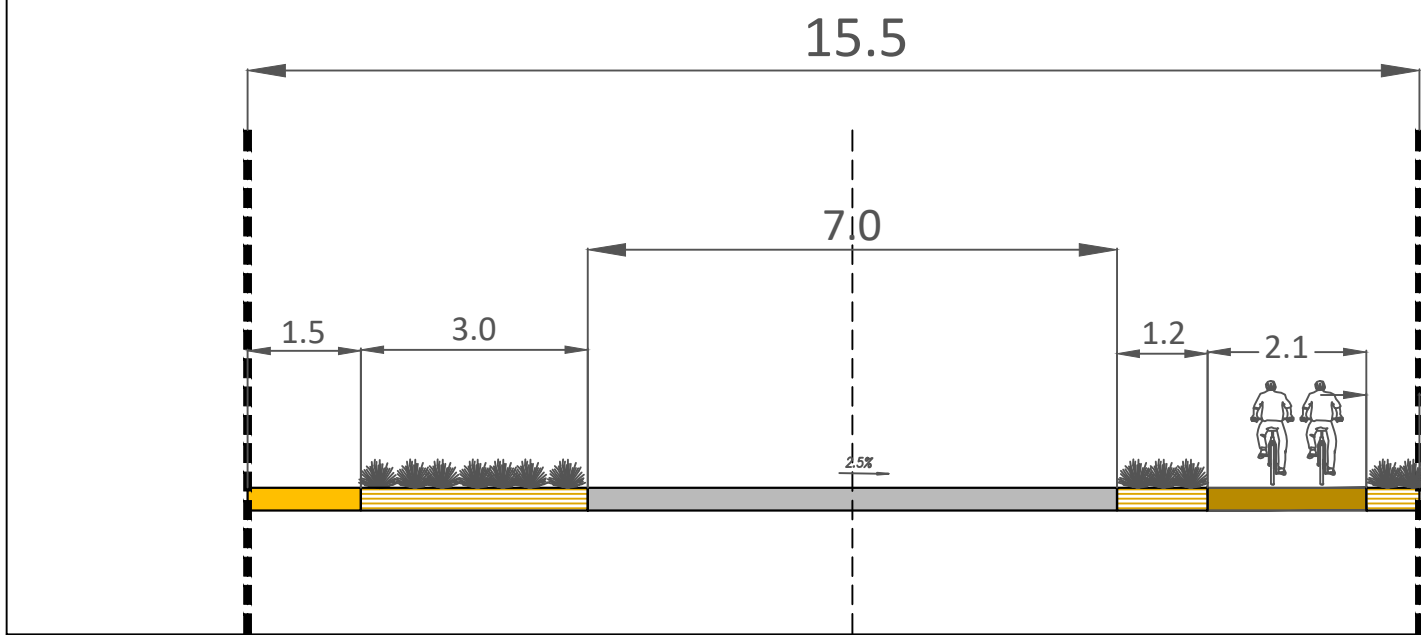
ПОПРЕЧНИ ПРОФИЛ 1-1
