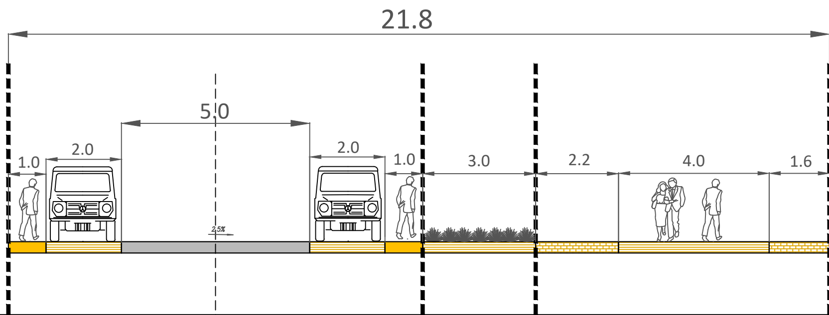
ПОПРЕЧНИ ПРОФИЛ 3-3
