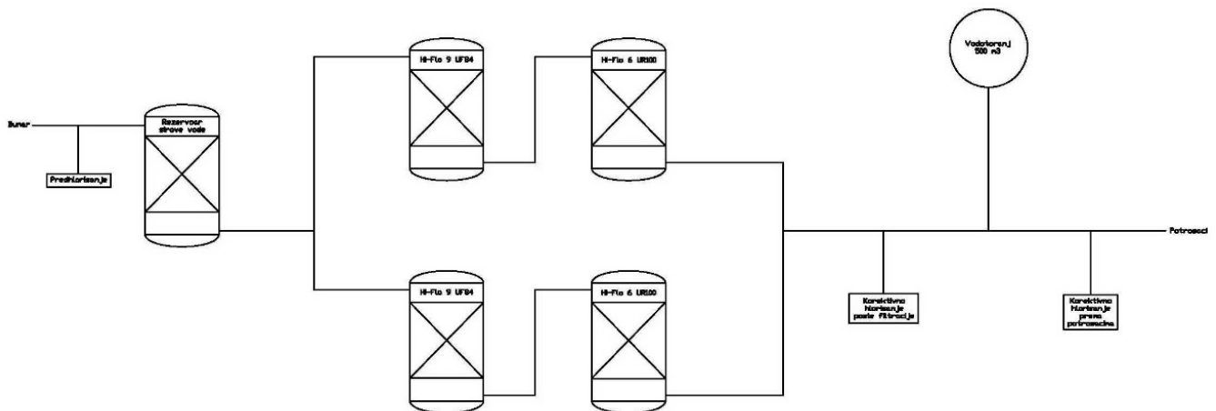
Сл. 1. Блок шема постројења за прераду воде за пиће на локацији ППВ Сонта
